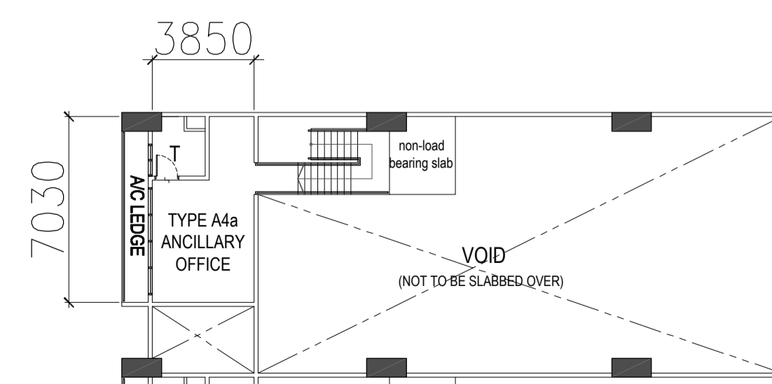
TYPE A4a - MEZZ STOREY PLAN
