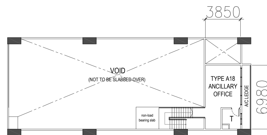
TYPE A18 - MEZZ STOREY PLAN
