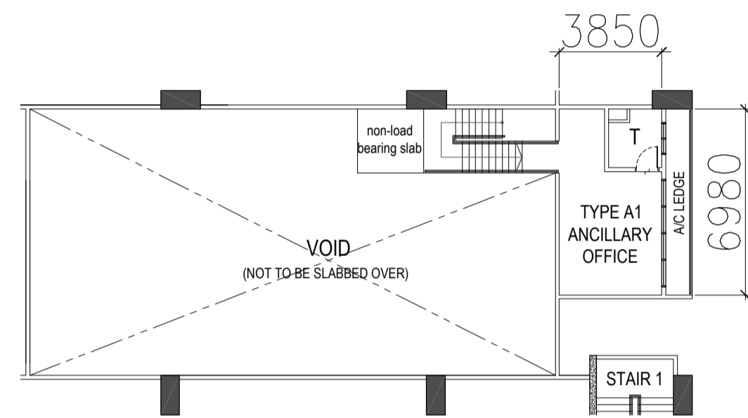
TYPE A1 - MEZZ STOREY PLAN
