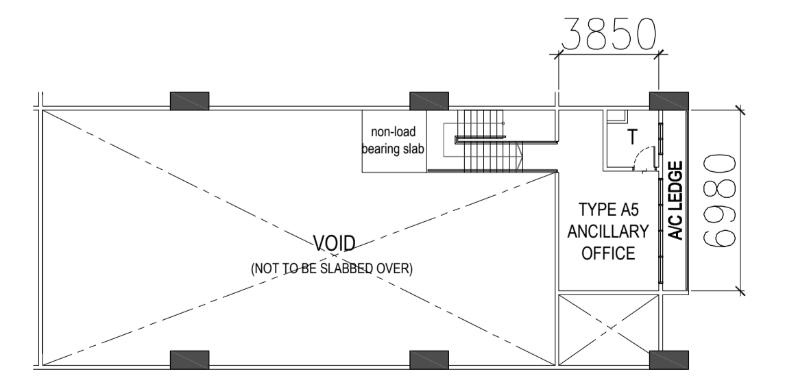
TYPE A5 - MEZZ STOREY PLAN
