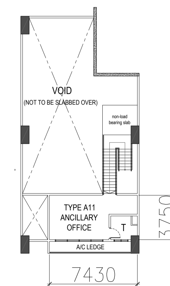
TYPE A11 - MEZZ STOREY PLAN
