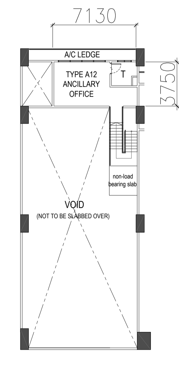
TYPE A12 - MEZZ STOREY PLAN
