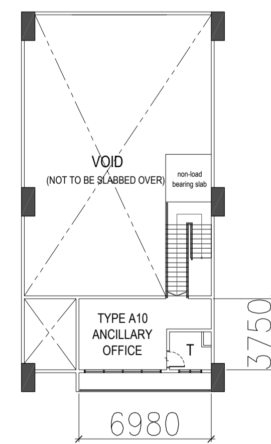
TYPE A10 - MEZZ STOREY PLAN
