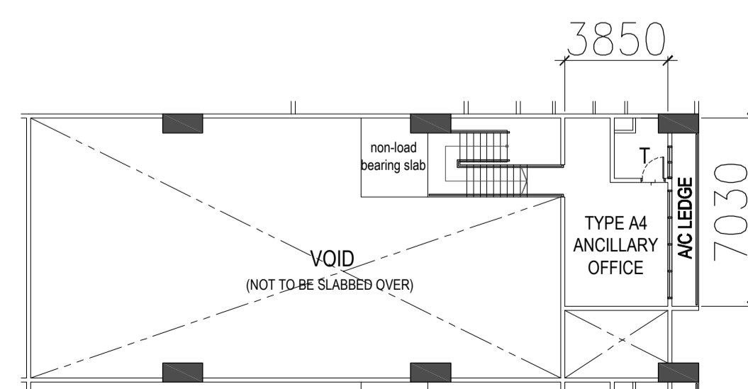
TYPE A4 - MEZZ STOREY PLAN
