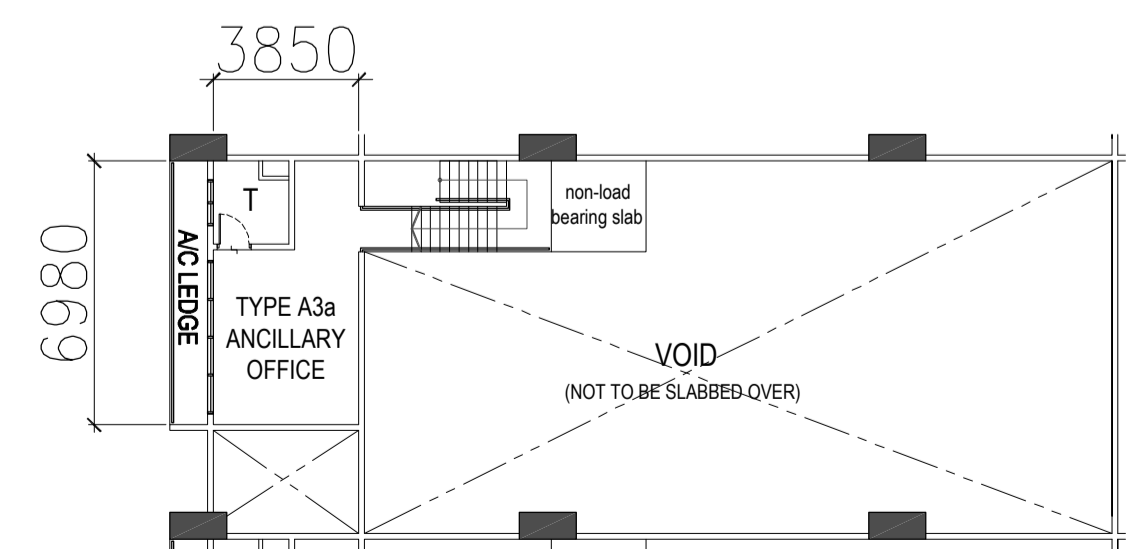
TYPE A3a - MEZZ STOREY PLAN
