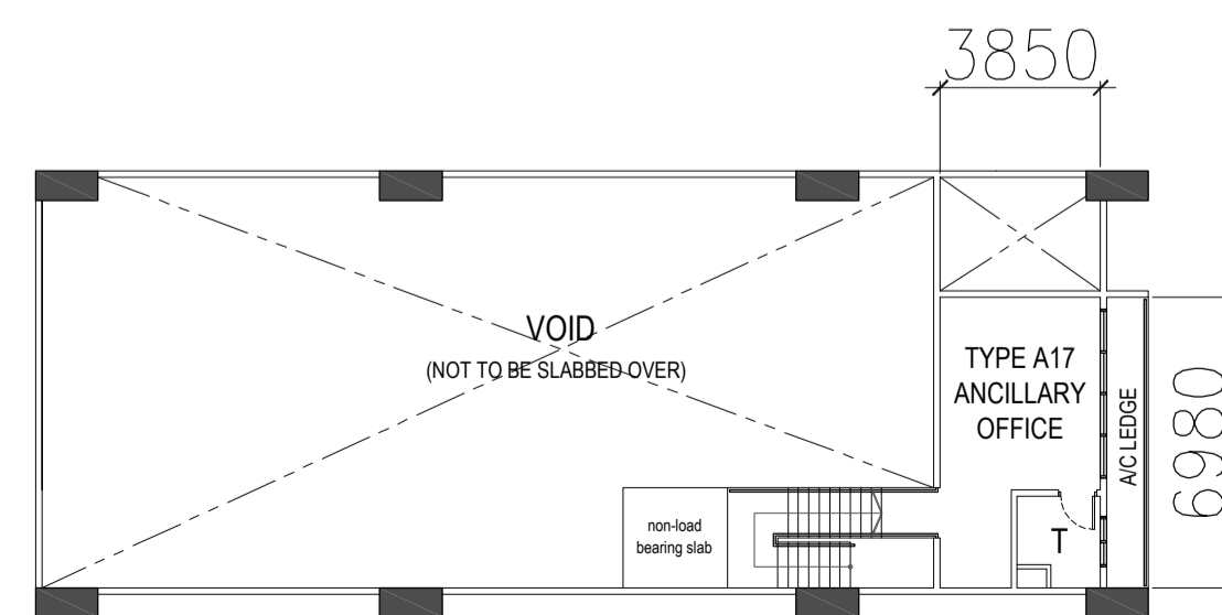
TYPE A17 - MEZZ STOREY PLAN
