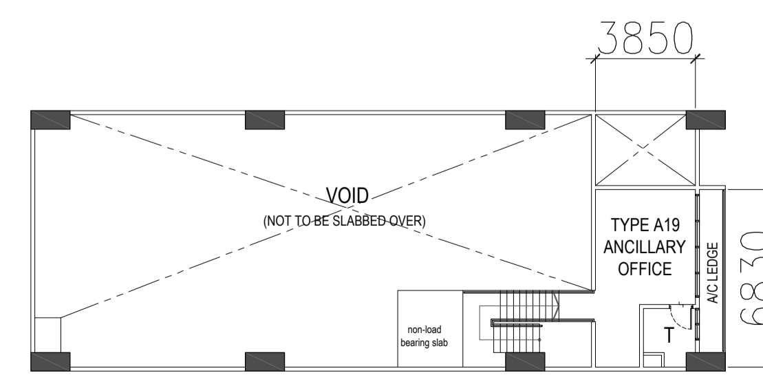
TYPE A19 - MEZZ STOREY PLAN
