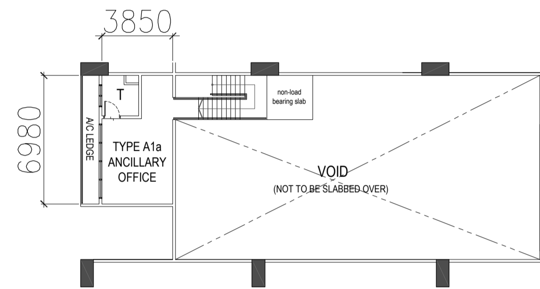
TYPE A1a - MEZZ STOREY PLAN
